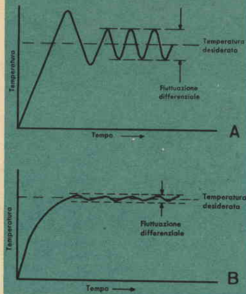
Fig. 3 - In A è illustrato il comportamento di un servomeccanismo discontinuo come un termostato acceso/aperto, mentre in B è illustrato il comportamento di un servosistema continuo come quello della fig. 2. La variazione di temperatura, o differenziale, è molto minore di quella che si ha in un sistema discontinuo.
