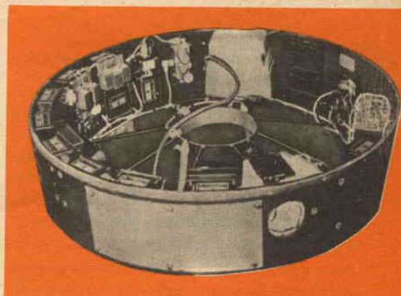
Il carico strumentale del razzo lunare « Pioneer » comprende dispositivi per la misura dei campi magnetici e della temperatura nell'interno del veicolo.
