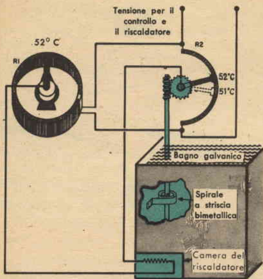
Fig. 2 Il bagno galvanico riscaldato illustra un servosistema continuo a circuito chiuso. Questo sistema controlla il calore con una precisione molto maggiore del termostato tipo acceso/aperto.
