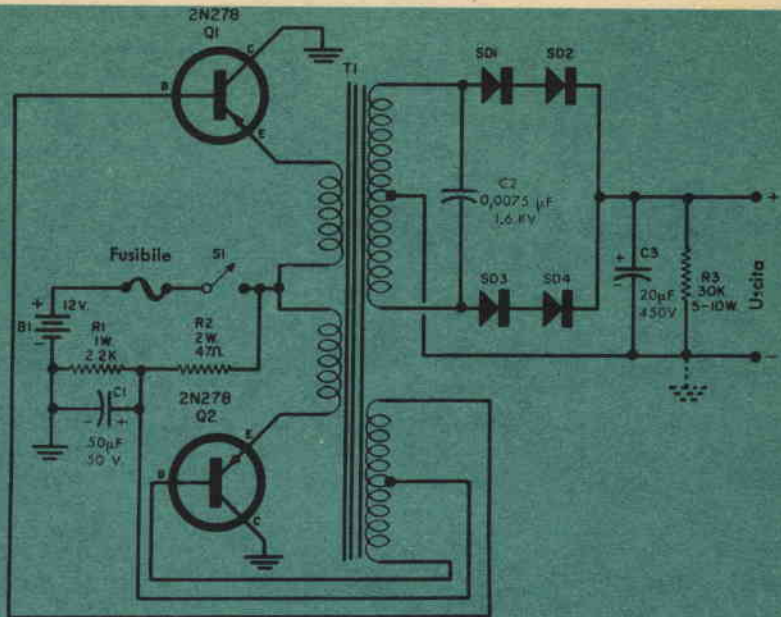
Fig. 2 - Alimentatore anodico a transistori per trasmettitori, ricevitori a onde corte, amplificatori e simili apparecchiature mobili.
