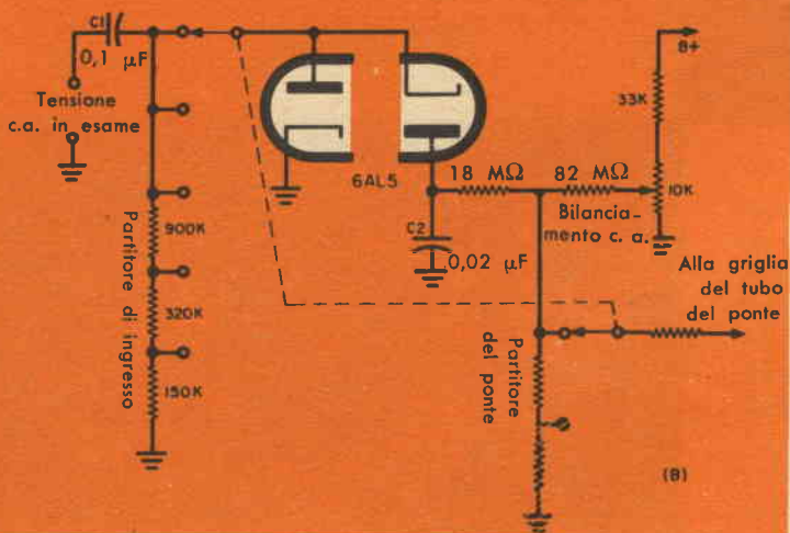
Fig. 2 - Due tipici raddrizzatori duplicatori di tensione usati nei voltmetri elettronici. I potenziali di contatto dei diodi si annullano a vicenda in A e il potenziometro di bilanciamento c.a. regola lo zero. In B il potenziale negativo viene annullato con una tensione prelevata dall'alimentatore e presente ai capi del potenziometro di bilanciamento.
